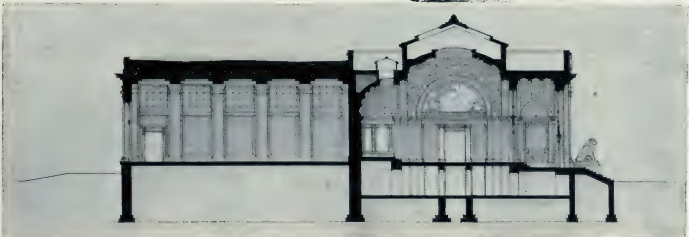
LONGITUDINAL SECTION.
